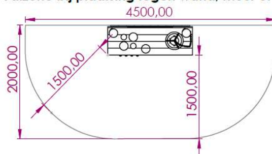
Valzone bij plaatsing tegen wand, muur of hek
